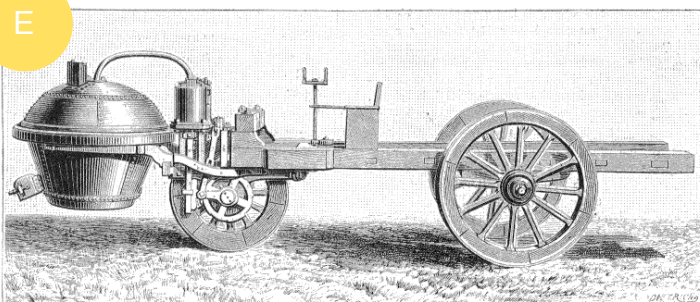
Fig. 1. — La première voiture à vapeur de Cugnot, expérimentée en 1770, actuellement exposée au Conservatoire des arts et métiers, à Paris.
